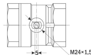
Вид А
