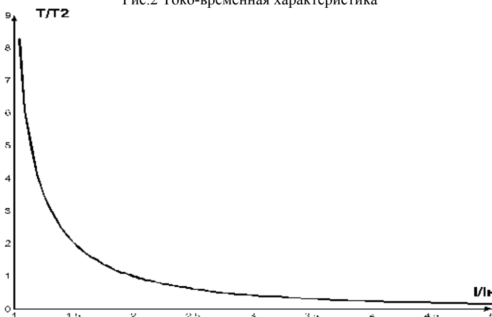
Рис.2 Токо-временная характеристика
