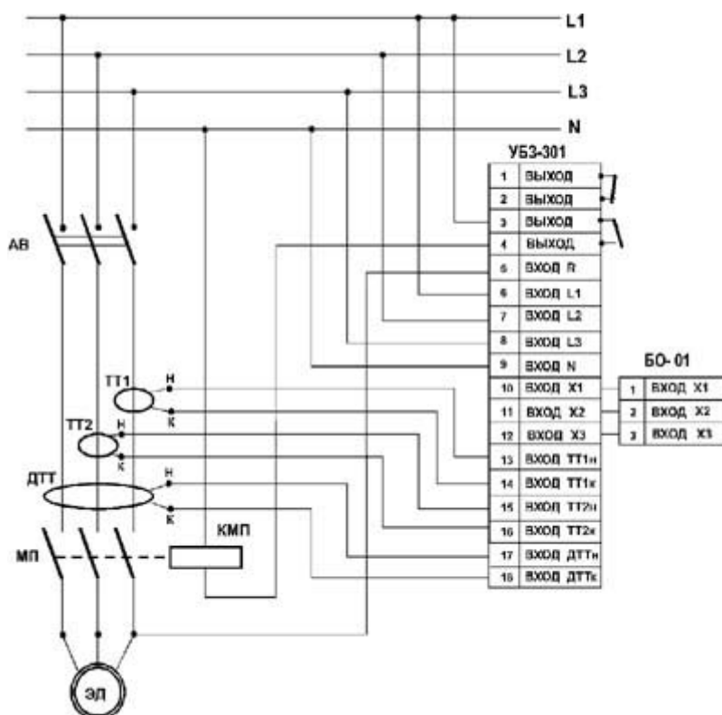
Схема подключения блока УБЗ-301
