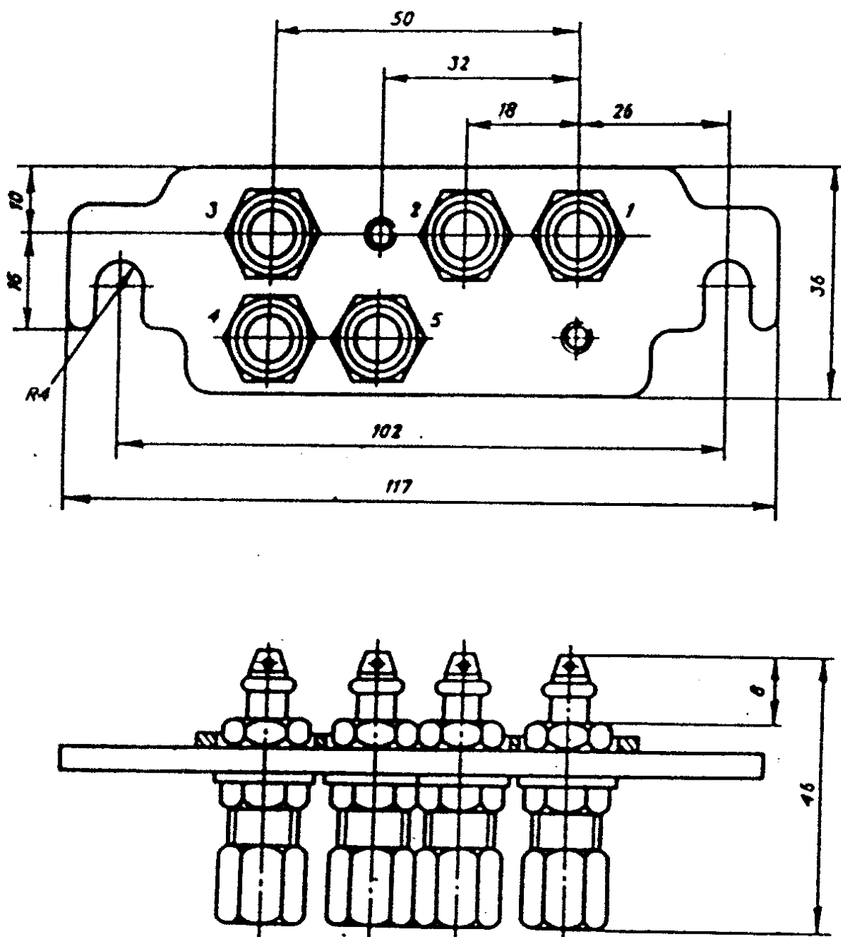
Рис. 9 Габаритные и установочные размеры вклн
