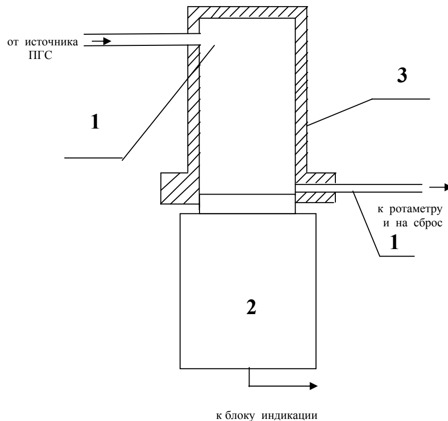
Рис. 3.1. Подача ПГС в адаптер при проверках
