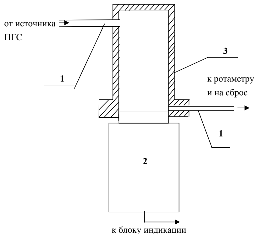
Рисунок 3.1 - Подача ПГС в адаптер при проверках 1 – соединительные трубки; 2 – блок датчиков; 3 – адаптер
