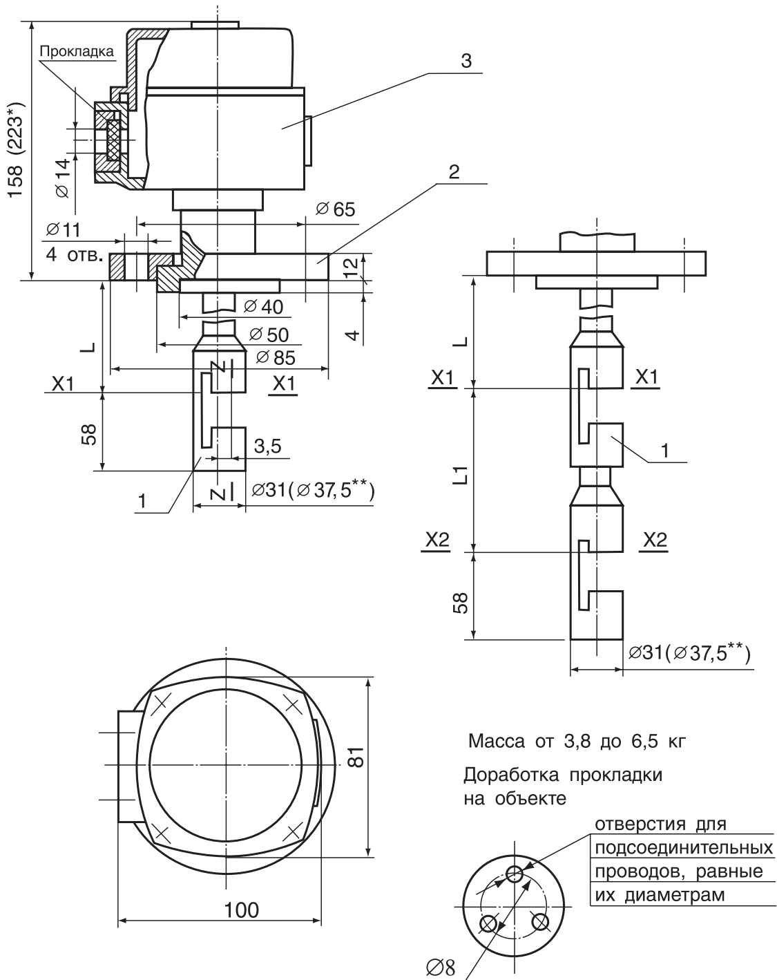
Датчики акустические АД-313(И), АД-323(И).
