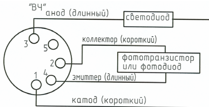
"ВЧ"-соединитель ОНЦ-ВГ-4-5/16-Р АШДК.434410.023 ТУ Светодиод - АЛ-107А ФЫО.336.015 ТУ Фототранзистор-ФТ-2К ТУЗ-3.1694-79 Рисунок Л1-Схема соединений "ВЧ" выхода счетчика газа СГ X1
