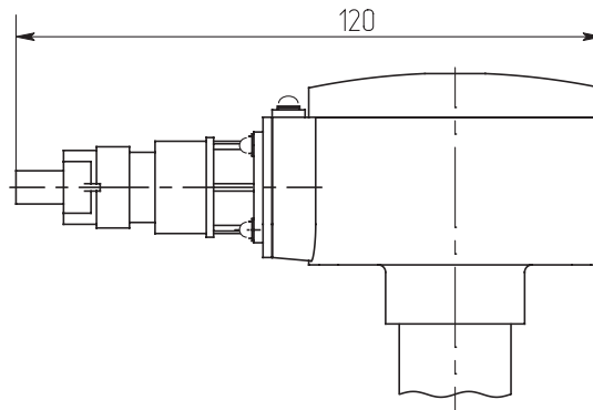
Габаритные размеры первичных преобразователей с разъемом ПП-212, ПП-216, ПП-225, ПП-264, ПП-266, ПП-292, ПП-293, ПП-294, ПП-295, ПП-296.
