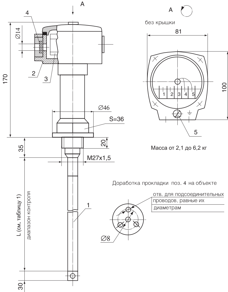
Преобразователь первичный ПП-296.
