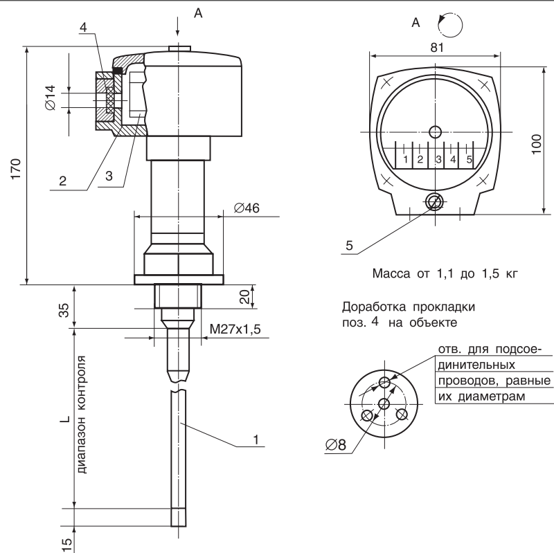
Преобразователь первичный ПП-025, 025И.
