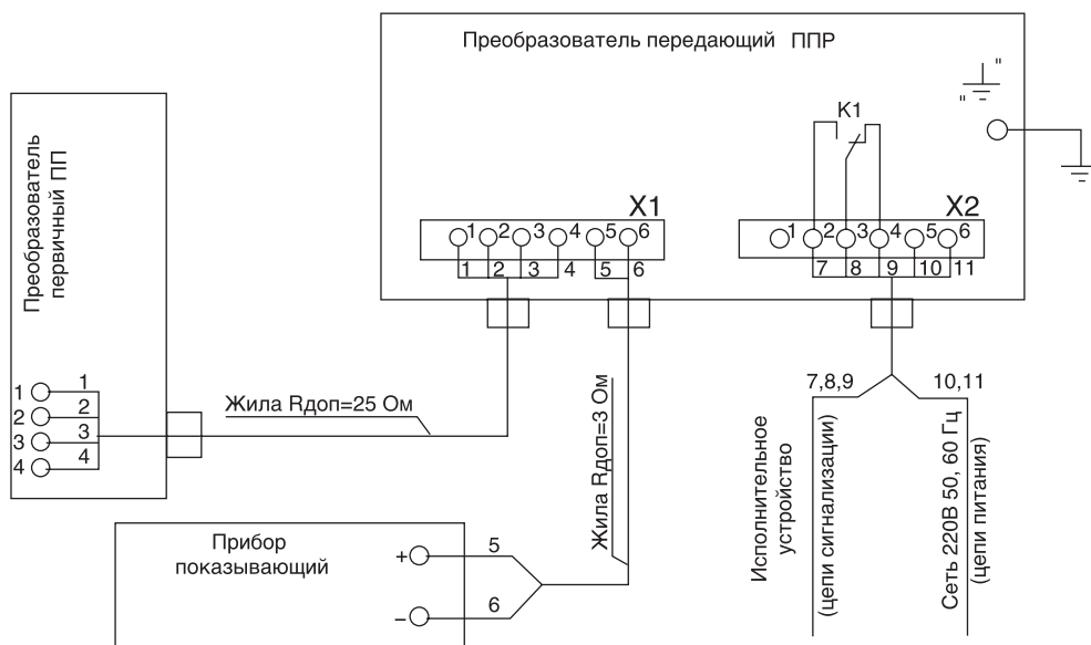
Схема электрическая подключения датчика-индикатора уровня РИС -101.
