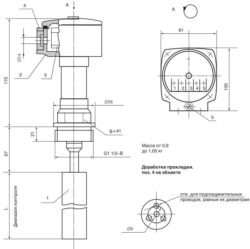
Преобразователь первичный ПП-016, 016И.
