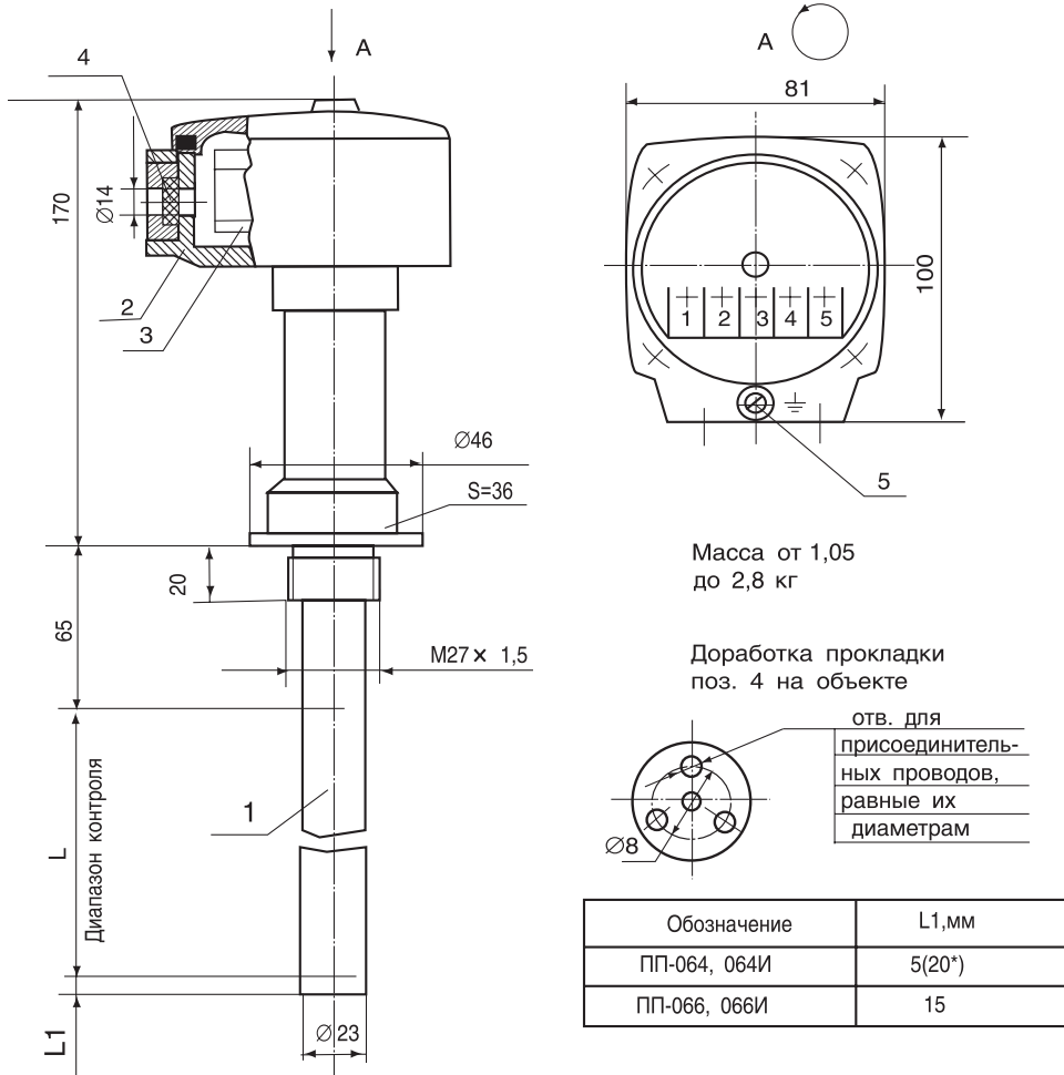
Преобразователь первичный ПП-064, ПП-066, 064И, 066И.
