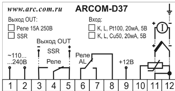
Рис.2. Схема подключения прибора.
