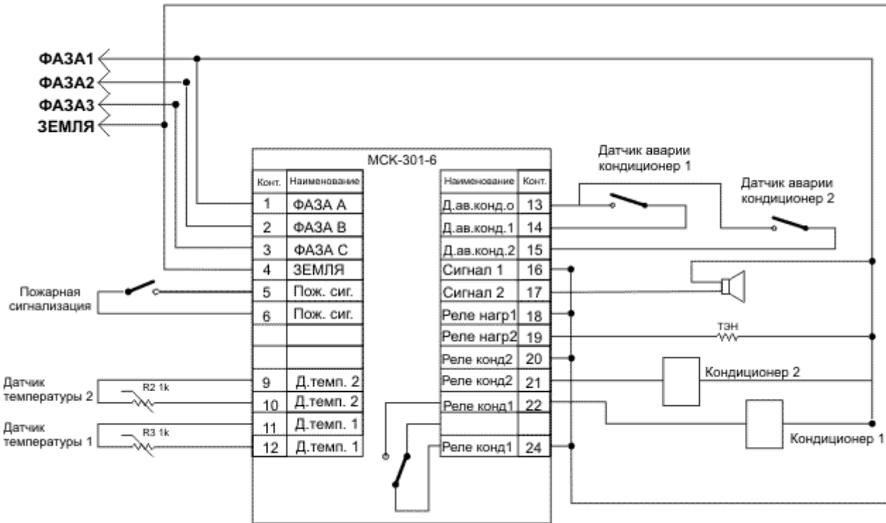
Рисунок 2. Схема подключения КУТП к трехфазной сети.
