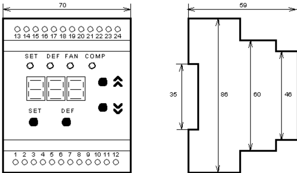
Рисунок 1. Лицевая панель, органы управления и габаритные размеры КУТП. Индикатор “COMP” горит, когда включен кондиционер №1. Индикатор “FAN” горит, когда включен кондиционер №2. Индикатор “DEF” горит, когда включен электронагреватель.
