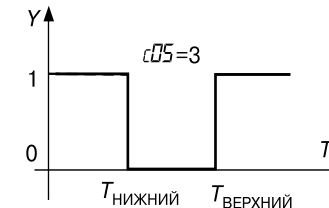
Рис. 17. Компаратор срабатывает вне установленных пределов
