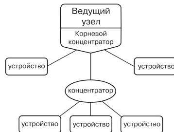
Рис. 1.2. Топология физической шины USB
