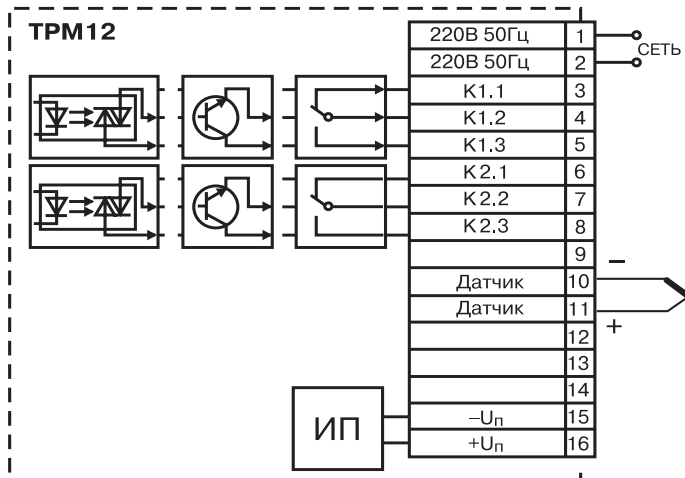
Рисунок Г.2. Схема подключения к приборам TPM12X термопар (для конструктивного исполнения "Н", "Щ1" и "Щ2")
