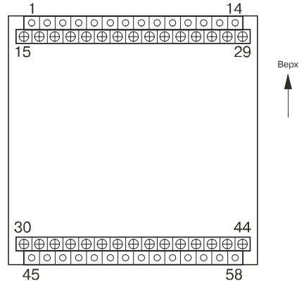
Рис. Б.1. Расположение клеммников на корпусе прибора
