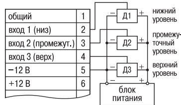
Рис. Б4. Схема подключения активных датчиков Д1...Д3 при питании их от внешнего источника
