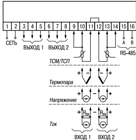
Рис. В.1. Общая схема подключения TRM202
