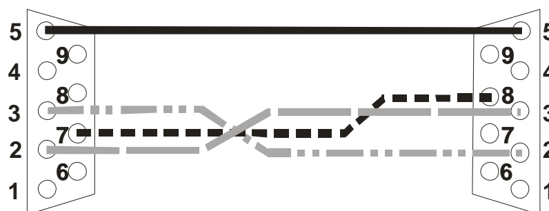
Рисунок 22. Схема нуль-модемного кабеля для программирования ИП320
