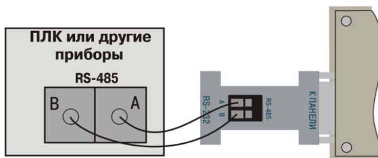
Рисунок 23. Схема подключения интерфейса RS-485 для конфигурирования панели ИП320
